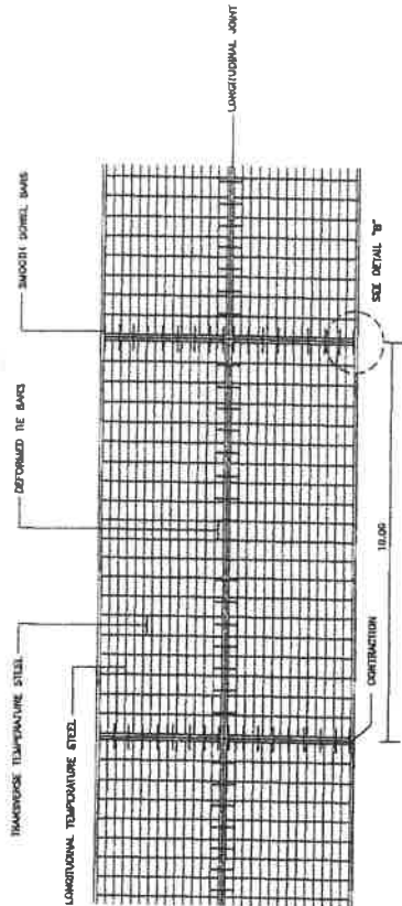
แบบแปลนการเสริมเหล็กแบบ ค.ร.ร.
